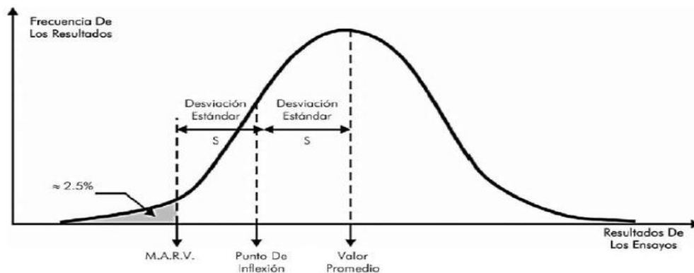
RELACIÓN RELATIVA DE LOS DIFERENTES VALORES USADOS EN LA ESPECIFICACIÓN DE LOS GEOTEXILES
